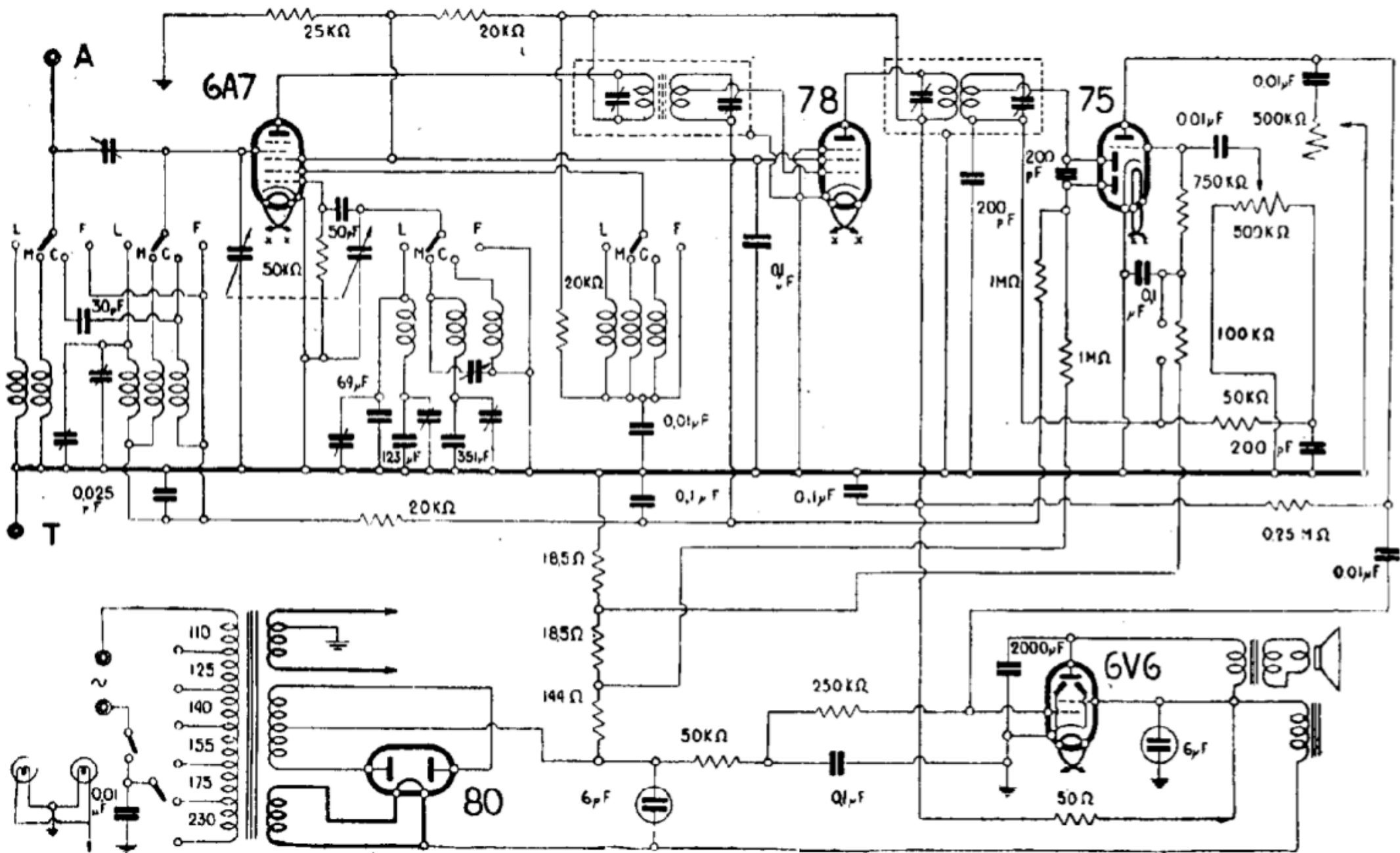
MAGNADYNE - MOD. « S 36 C »
